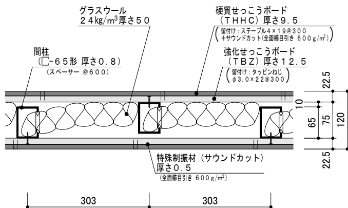
水平断面图
