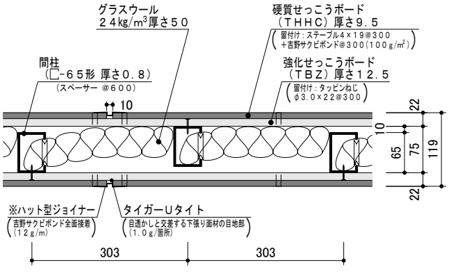
水平断面図
