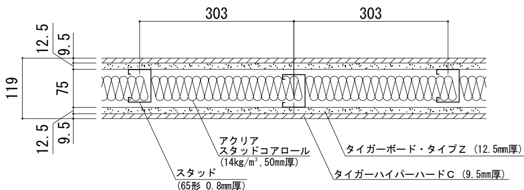
水平断面図（「ハイパーウォールZ・W I アクリア仕様」遮音測定時（S-247-27参照）の壁構造）
